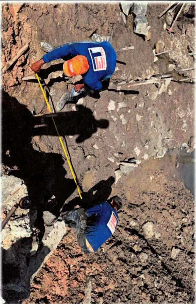
Foto n. 17 CONCRETO MAGRO PARA LASTRO
