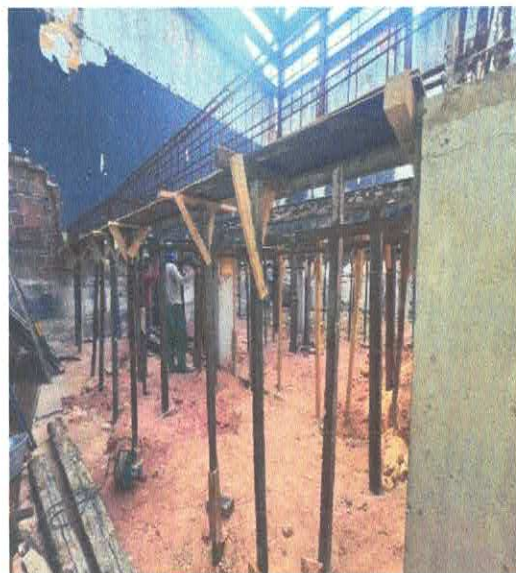
FOTO 18: ARMAÇÃO DE LAJE DE ESTRUTURA CONVENCIONAL DE CONCRETO ARMADO UTILIZANDO AÇO CA-50 DE 6,3 MM.
