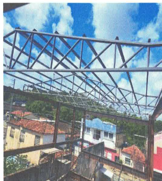
FOTO 20: ESTRUTURA TRELIÇADA DE COBERTURA, TIPO FINK, COM LIGAÇÕES SOLDADAS, INCLUSOS PERFIS METÁLICOS, CHAPAS METÁLICAS, MÃO DE OBRA E TRANSPORTE COM GUINDASTE.
