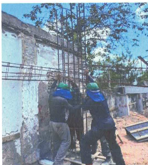
FOTO 11: ARMAÇÃO DE PILAR OU VIGA DE ESTRUTURA CONVENCIONAL DE CONCRETO ARMADO UTILIZANDO AÇO CA-50 DE 6,3 MM.
