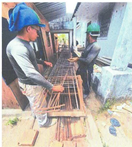
FOTO 07: ARMAÇÃO DE PILAR OU VIGA DE ESTRUTURA CONVENCIONAL DE CONCRETO ARMADO UTILIZANDO AÇO CA-50 DE 20,0 MM.
