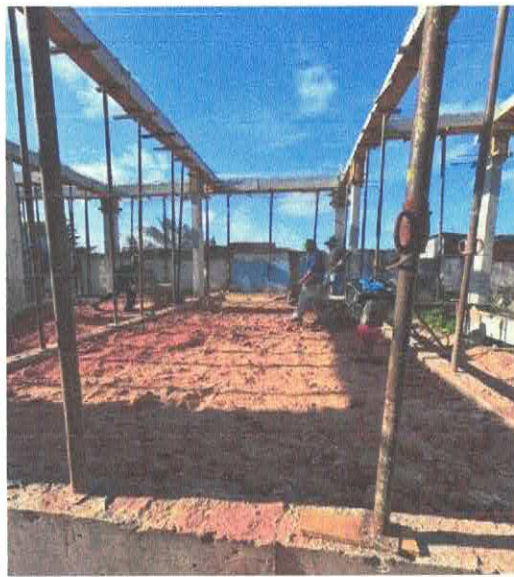
FOTO 02: ATERRO MANUAL DE VALAS COM AREIA PARA ATERRO E COMPACTAÇÃO MECANIZADA.
