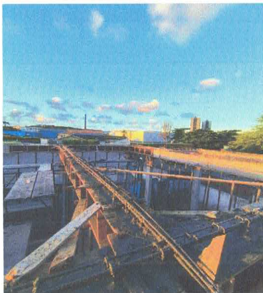
FOTO 09: CONCRETO SIMPLES USINADO FCK=35MPA, BOMBEADO, LANÇADO E ADENSADO EM SUPERESTRUTURA.
