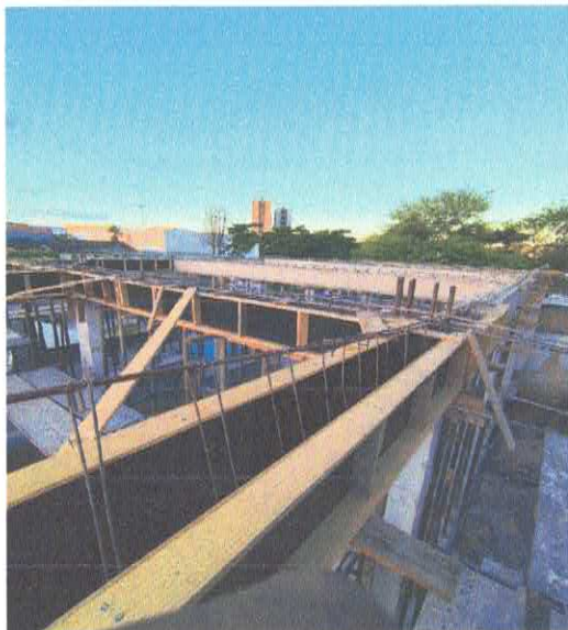
FOTO 17: ARMAÇÃO DE LAJE DE ESTRUTURA CONVENCIONAL DE CONCRETO ARMADO UTILIZANDO AÇO CA-50 DE 12,5 MM.
