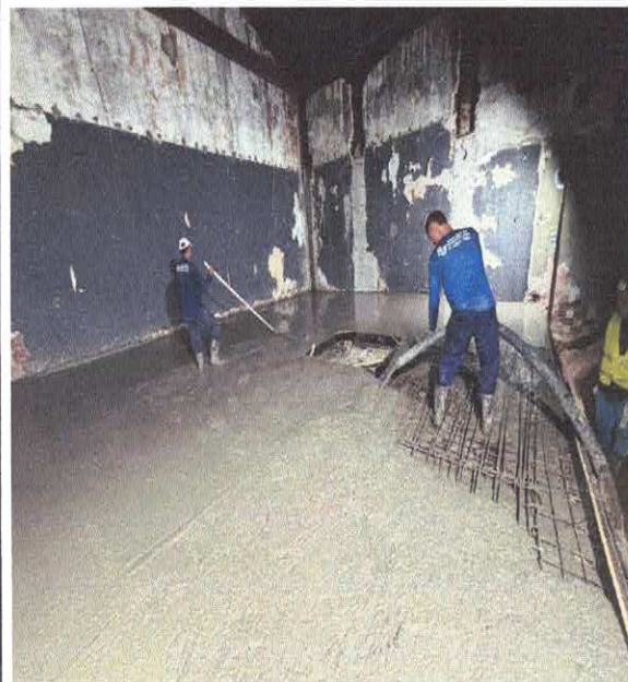
FOTO 13: COMP. 113 - Concreto simples usinado f_{ck}=35\text{mpa} , bombeado, lançado e adensado em superestrutura.
