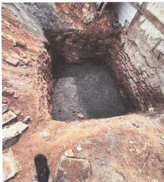
FOTO 03: COMP. 111 - SOLO-CIMENTO COMPACTADO - TRAÇO 1:20, INCLUSIVE CIMENTO E AREIA.
