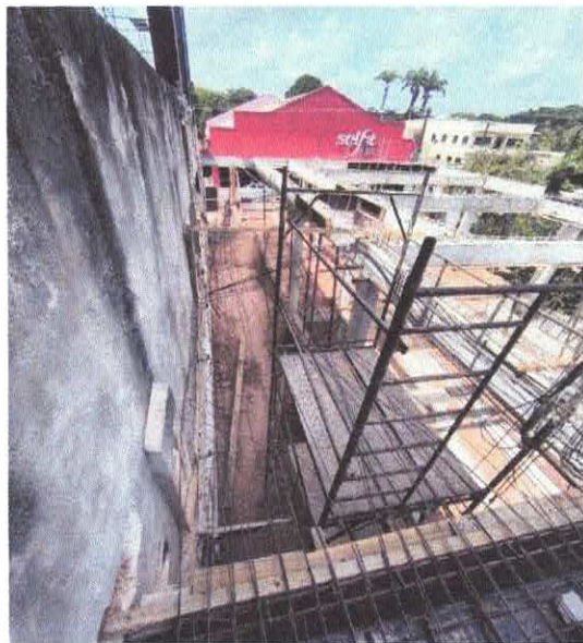
FOTO 17: MONTAGEM E DESMONTAGEM DE ANDAIME MODULAR FACHADEIRO, COM PISO METÁLICO, PARA EDIFICAÇÕES COM MÚLTIPLOS PAVIMENTOS.
