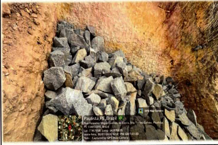
Foto nº08 6.2.3. - ALVENARIA EM PEDRA RACHÃO OU PEDRA DE MÃO, ASSENTADA COM ARGAMASSA TRACO 1:6 (CIMENTO E AREIA)
