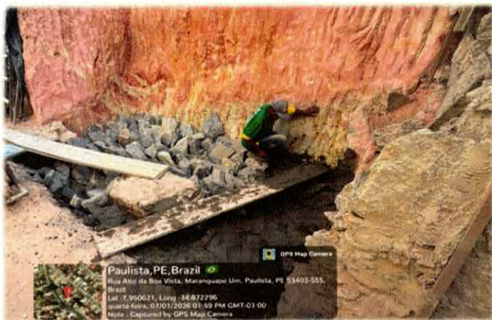
Foto n10 1.2.11. - ALVENARIA EM PEDRA RACHÃO OU PEDRA DE MÃO, ASSENTADA COM ARGAMASSA TRACO 1:6
