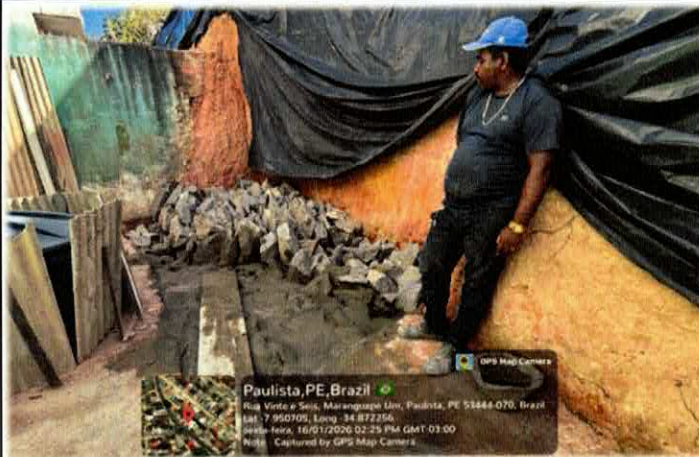
Foto n11 1.2.11. - ALVENARIA EM PEDRA RACHÃO OU PEDRA DE MÃO, ASSENTADA COM ARGAMASSA TRACO 1:6
