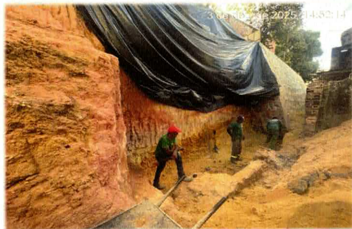
Foto n13 1.2.3. - REGULARIZAÇÃO E COMPACTAÇÃO DE TERRENO, COM SOQUETE
