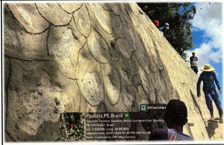
Foto n. 04 EXECUÇÃO DE MURO DE CONTENÇÃO EM ALVENARIA DE PEDRA RACHÃO, COM TRAÇO DE ARGAMASSA.
