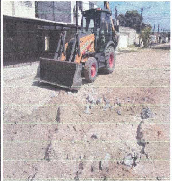
FOTO 18: REATERRO MECANIZADO DE VALA COM ESCAVADEIRA HIDRÁULICA (CAPACIDADE DA CAÇAMBA: 0,8 M³ / POTÊNCIA: 111 HP)
