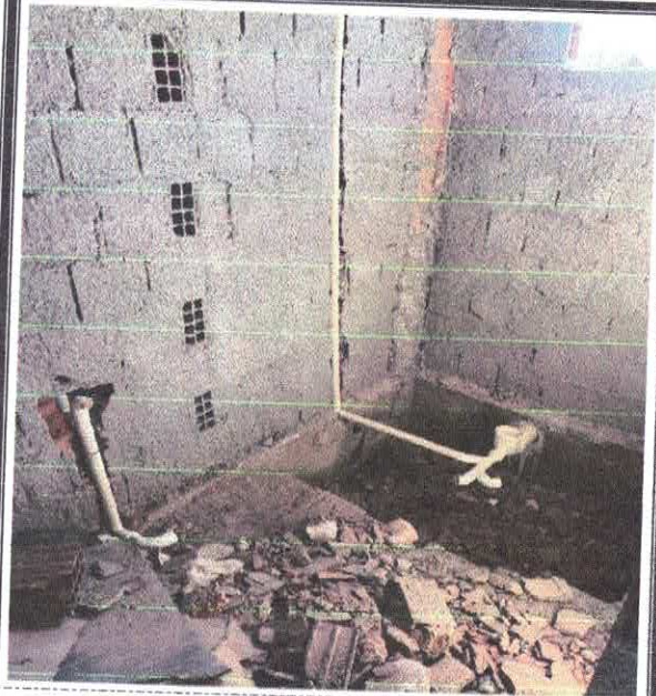
FOTO 14: CAIXA SIFONADA, PVC, DN 100 X 100 X 50 MM, FORNECIDA E INSTALADA EM RAMAIS DE ENCAMINHAMENTO DE ÁGUA PLUVIAL. AF_06/2022
