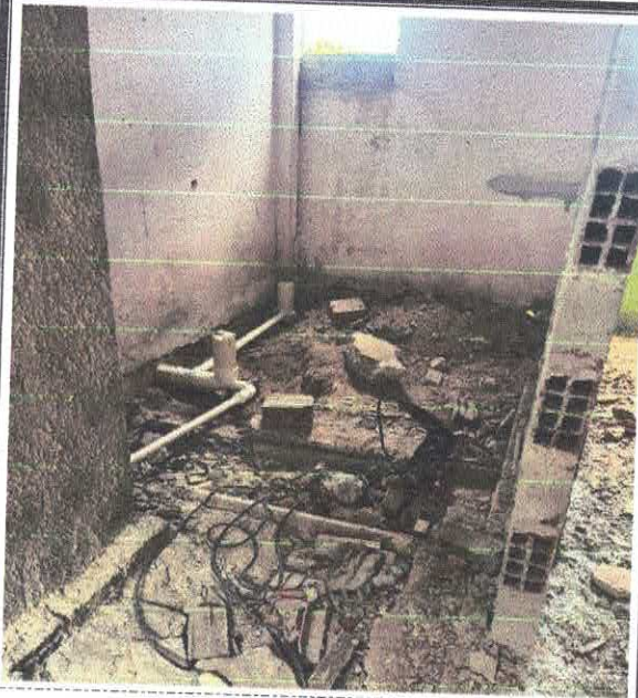
FOTO 13: PONTO DE ESGOTO PARA BACIA SANITÁRIA, INCLUSIVE TUBULAÇÕES E CONEXÕES EM PVC RÍGIDO SOLDÁVEIS, ATÉ A COLUNA OU O SUB-COLETOR.
