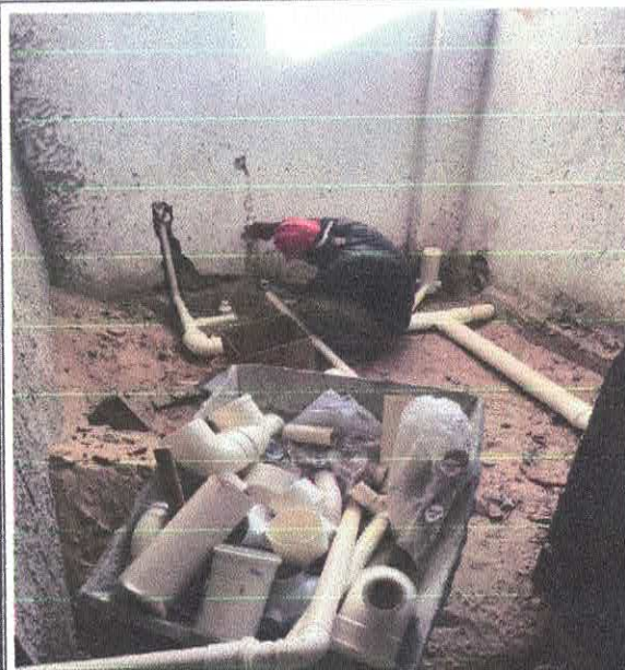
FOTO 12: TUBO PVC, SERIE NORMAL, ESGOTO PREDIAL, DN 50 MM, FORNECIDO E INSTALADO EM RAMAL DE DESCARGA OU RAMAL DE ESGOTO SANITÁRIO. AF_08/2022
