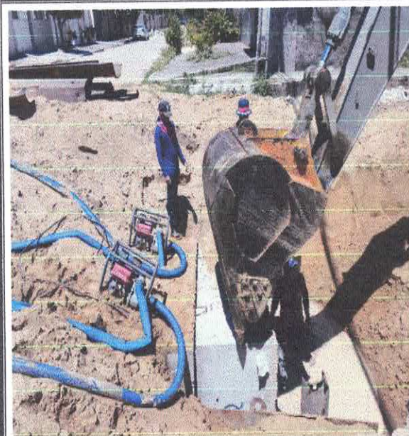
FOTO 23: ESGOTAMENTO COM BOMBA CENTRÍFUGA MONOESTÁGIO COM MOTOR ELÉTRICO O A COMBUSTÃO CHP DIURNO
