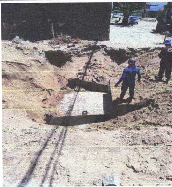
FOTO 21: ESCORAMENTO DE VALAS COM PRANCÕES METÁLICOS - ÁREA NÃO CRAVADA
