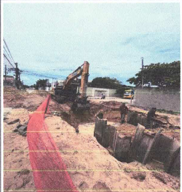
FOTO 20: ESCORAMENTO DE VALAS COM PRANCHOES METALICOS - AREA CRAVADA
