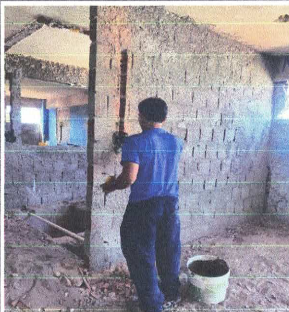
FOTO 08: CHAPISCO APLICADO EM ALVENARIAS E ESTRUTURAS DE CONCRETO INTERNAS, COM COLHER DE PEDREIRO. ARGAMASSA TRAÇO 1:3 COM PREPARO MANUAL. AF_10/2022
