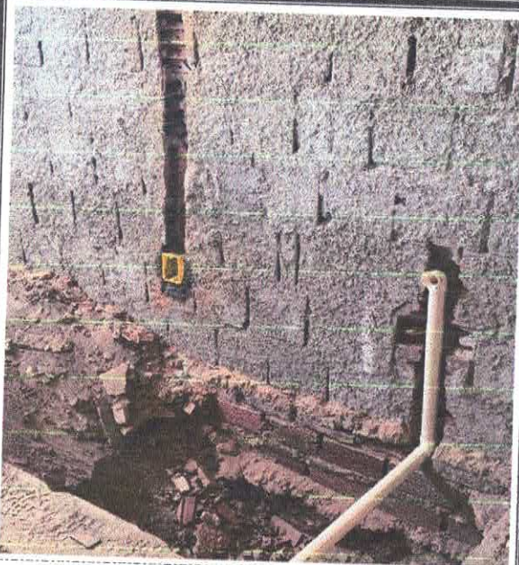
FOTO 15: PONTO DE ESGOTO PARA LAVATÓRIO OU MICTÓRIO, INCLUSIVE TUBULAÇÕES E CONEXÕES EM PVC RÍGIDO SOLDÁVEIS, ATÉ A COLUNA OU O SUB-COLETOR
