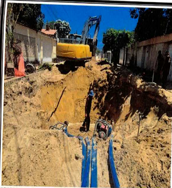
FOTO 06: ESGOTAMENTO COM BOMBA CENTRÍFUGA MONOESTÁGIO COM MOTOR ELÉTRICO O A COMBUSTÃO CHP DIURNO.
