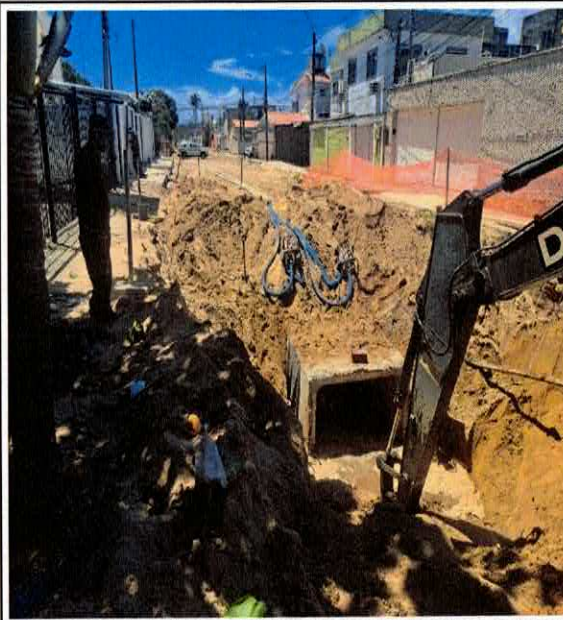
FOTO 02: ESCAVAÇÃO MECÂNICA DE VALAS (SOLO COM ÁGUA), PROFUNDIDADE MAIOR QUE 1,5 A 4,00 M.
