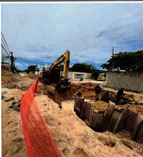
FOTO 01: ESCAVAÇÃO MECANIZADA DE VALA COM PROF. MAIOR QUE 1,5 M ATÉ 3,0 M COM ESCAVADEIRA, EM SOLO DE 2ª CATEGORIA, EM LOCAIS COM ALTO NÍVEL DE INTERFERÊNCIA.
