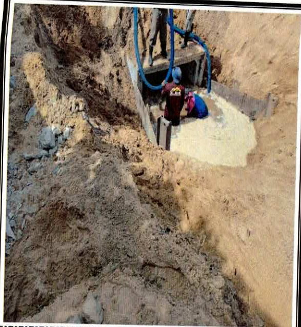
FOTO 05: ESCORAMENTO DE VALAS COM PRANCÕES METÁLICOS - ÁREA CRAVADA.
