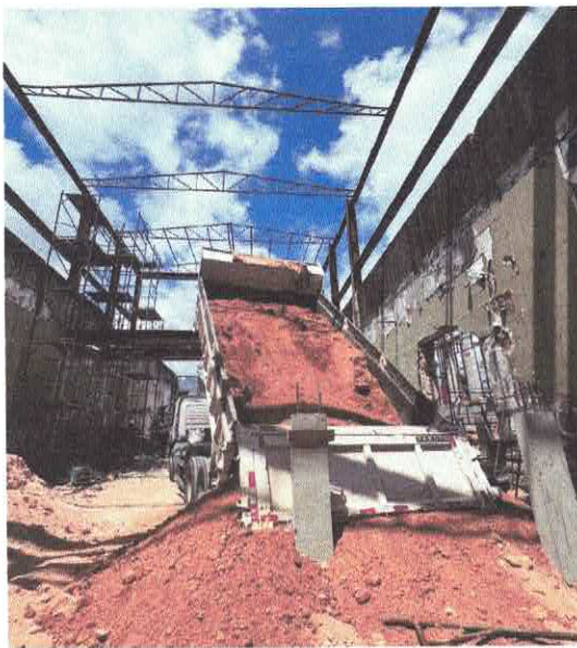
FOTO 09: ATERRO MANUAL DE VALAS COM AREIA PARA ATERRO E COMPACTAÇÃO MECANIZADA.
