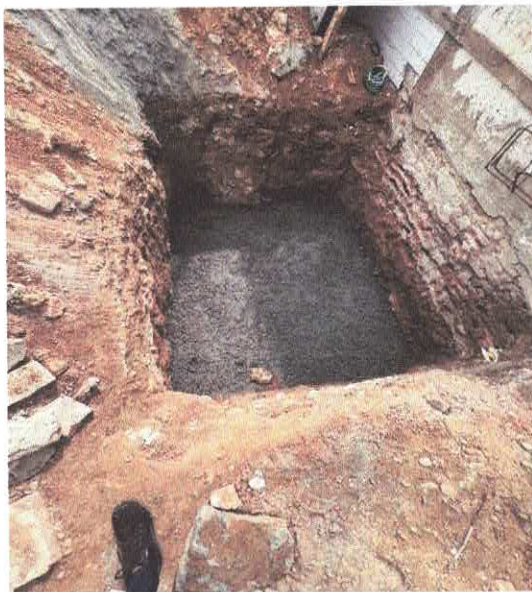
FOTO 11: COMP. 114 - LASTRO DE CONCRETO, FCK=15 MPA, LANÇADO E ADENSADO.
