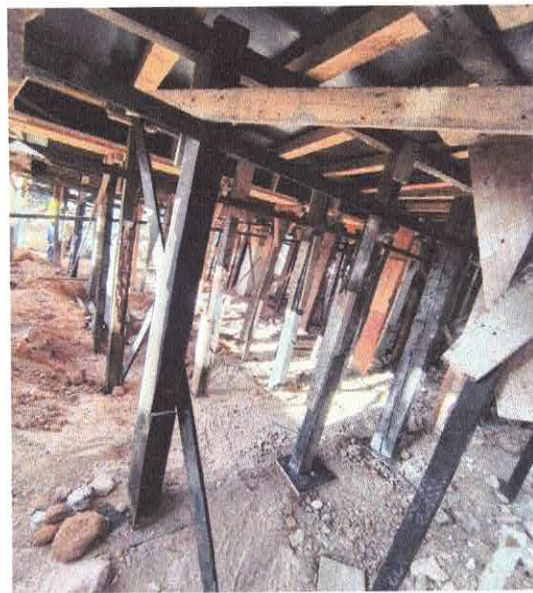
FOTO 20: COMP. 292 - FABRICAÇÃO E INSTALAÇÃO DE ESCORAS DE VIGA, EM MADEIRA. AF_09/2020.
