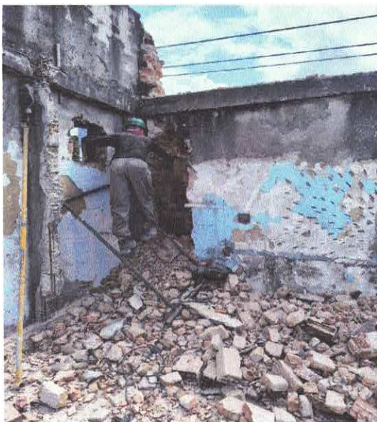
FOTO 05: DEMOLIÇÃO DE LAJES, DE FORMA MECANIZADA COM MARTELETE, SEM REAPROVEITAMENTO.
